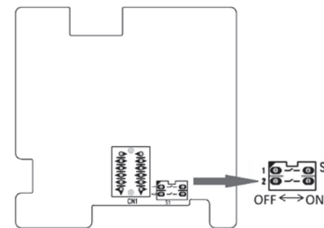
Рис. 28. Схема DIP-переключателей
